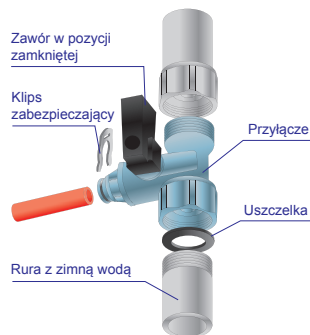
Rys.3. Przyłącze wody
